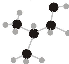
isobutyl alcohol \text{CH}_3-\text{CH}(\text{CH}_3)-\text{CH}_2-\text{OH}
