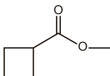
Ester (1)
