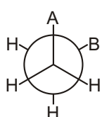
'gauche effect'
