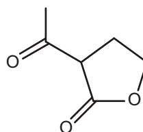
Ester, ketone (3)
