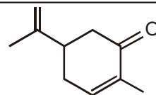
Carvone
